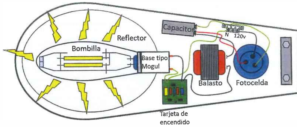
Diagrama de Luminaria con sus Componentes
